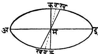
ध्रुवांचे चलन दाखविणारी आकृति.
